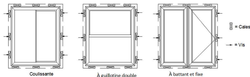
Figure 2 Emplacement des cales et des vis
