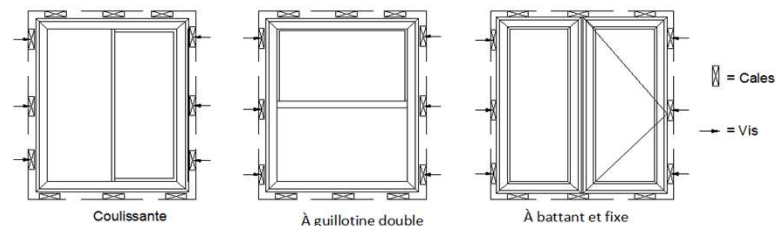
Figure 3 Emplacement des cales et des vis
