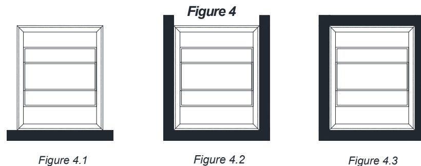
Méthode de solin
