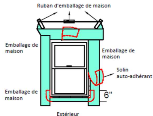
Méthode de solin
